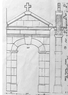
Projet de la porte d'entrée du côté paroisse
